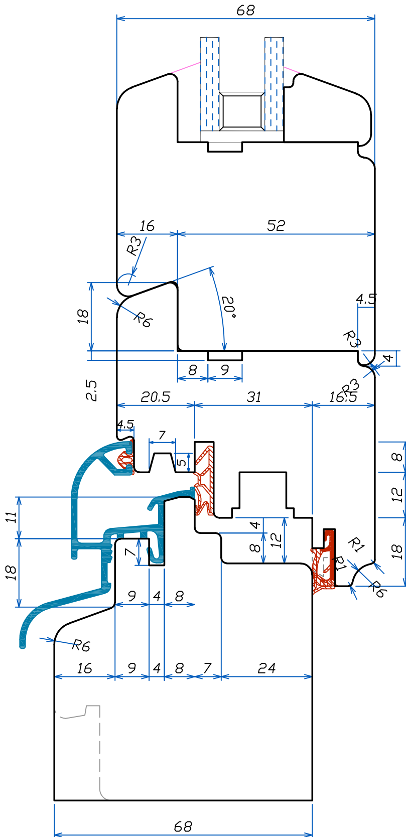
SEZIONE VERTICALE FINESTRA
