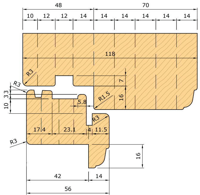
Sezione verticale Vertical section
