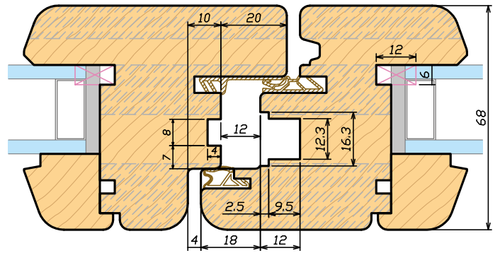
Sezione orizzontale - Chiusura centrale 68 Horizontal section - Central closure 68
