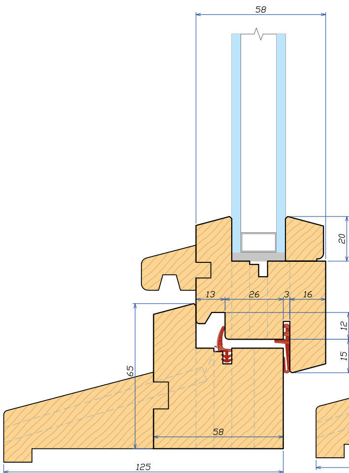
Sezione verticale 58 Vertical section 58
