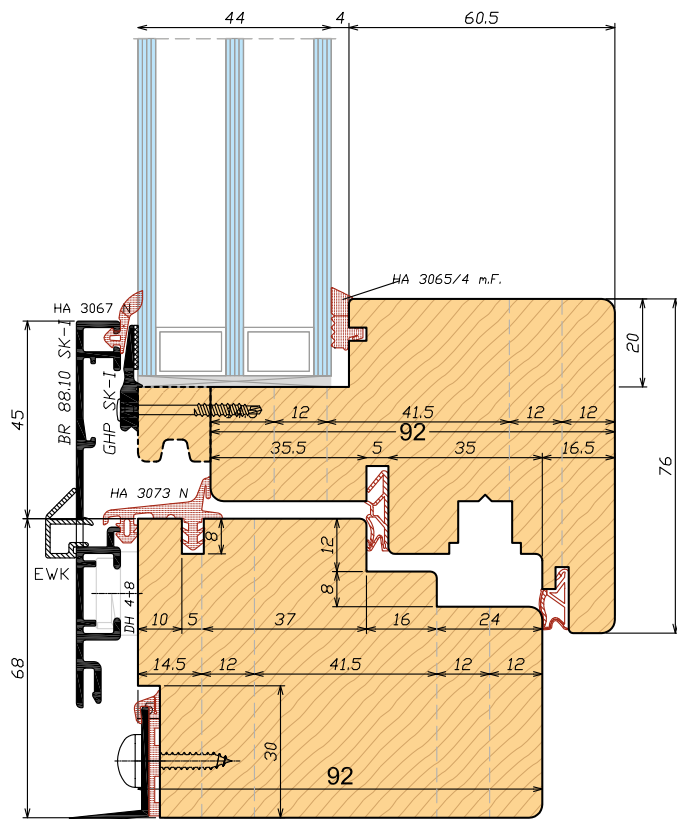
Sezione verticale Vertical section
