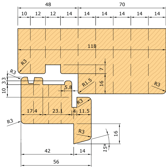
Sezione verticale Vertical section
