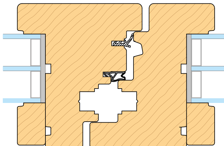
Sezione orizzontale - Chiusura centrale Horizontal section - Central closure
