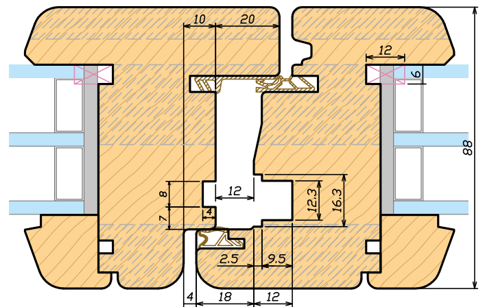
Sezione orizzontale - Chiusura centrale 88 Horizontal section - Central closure 88
