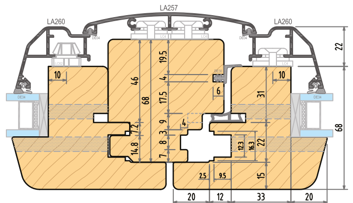
Montantino aggiuntivo Additional jamb
