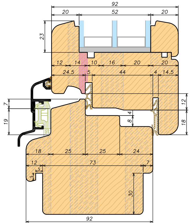
Sezione orizzontale - Chiusura centrale 92 Horizontal section - Central closure 92
