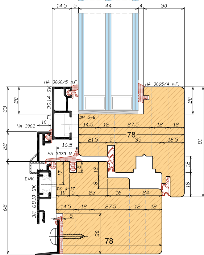
Sezione verticale Vertical section
