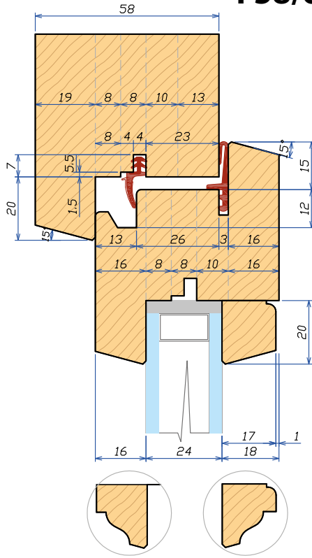
Sezione verticale 58 Vertical section 58
