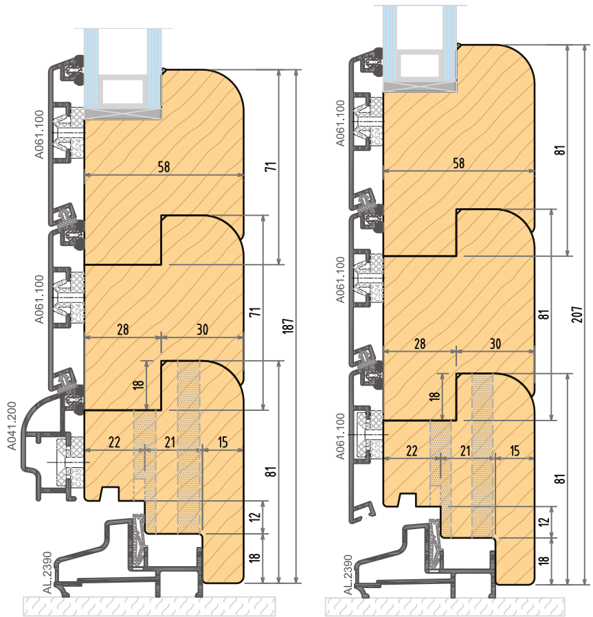
Sezione verticale - Portafinestra Vertical section - French door
