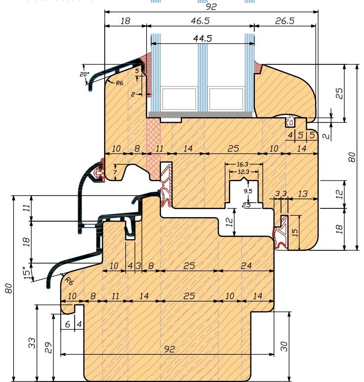
Sezione orizzontale - Chiusura centrale 92 Horizontal section - Central closure 92
