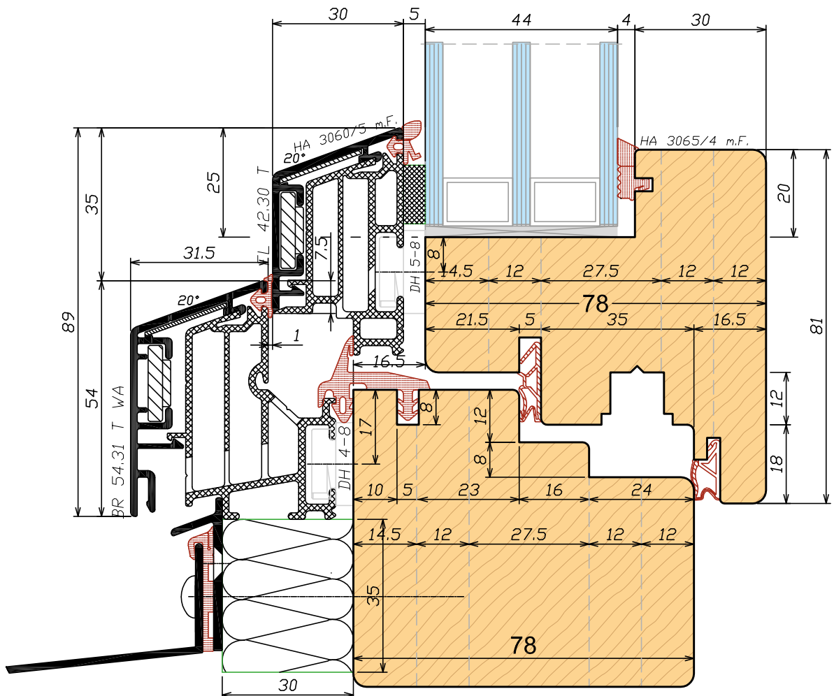
Sezione verticale Vertical section
