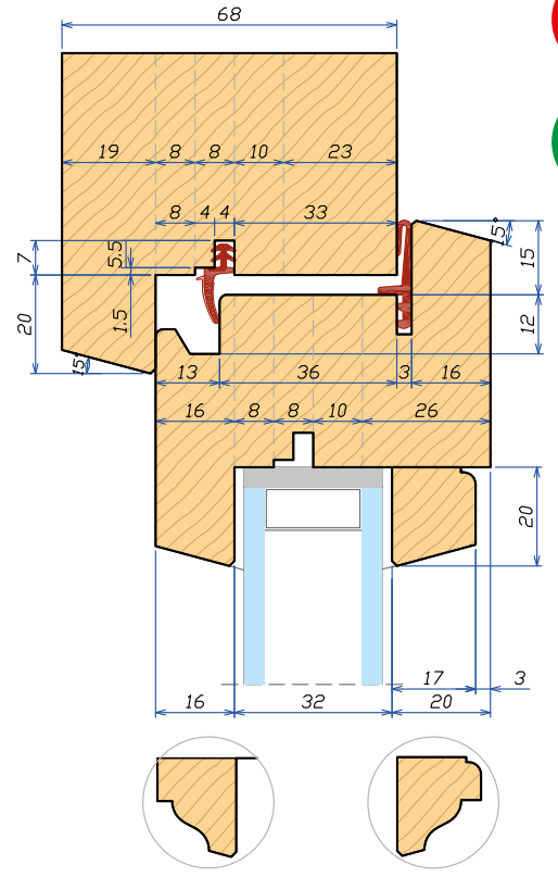
Sezione verticale 68 Vertical section 68
