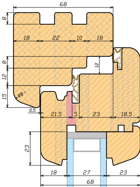
Sezione verticale 68 Vertical section 68
