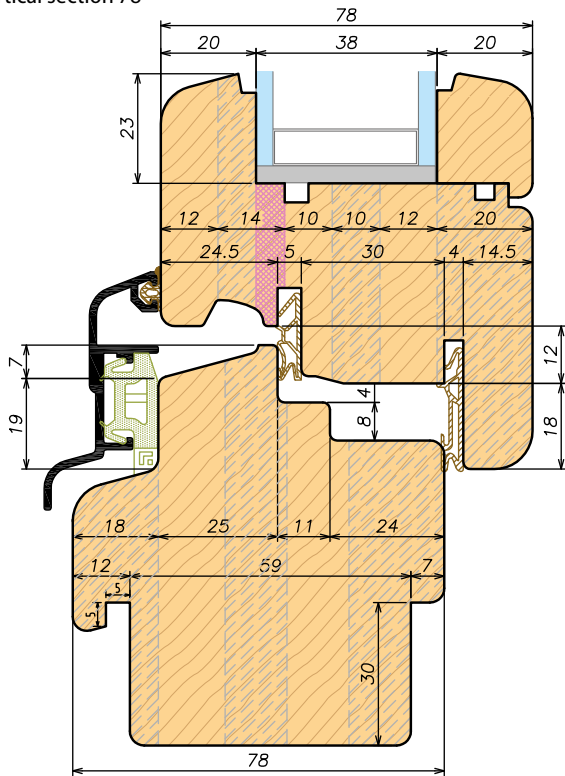
Sezione orizzontale - Chiusura centrale 78 Horizontal section - Central closure 78
