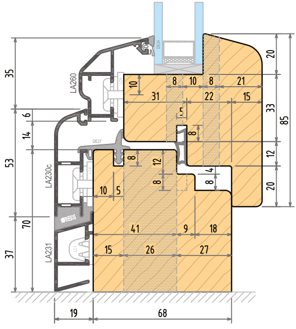
Sezione orizzontale chiusura centrale Horizontal section central closure
