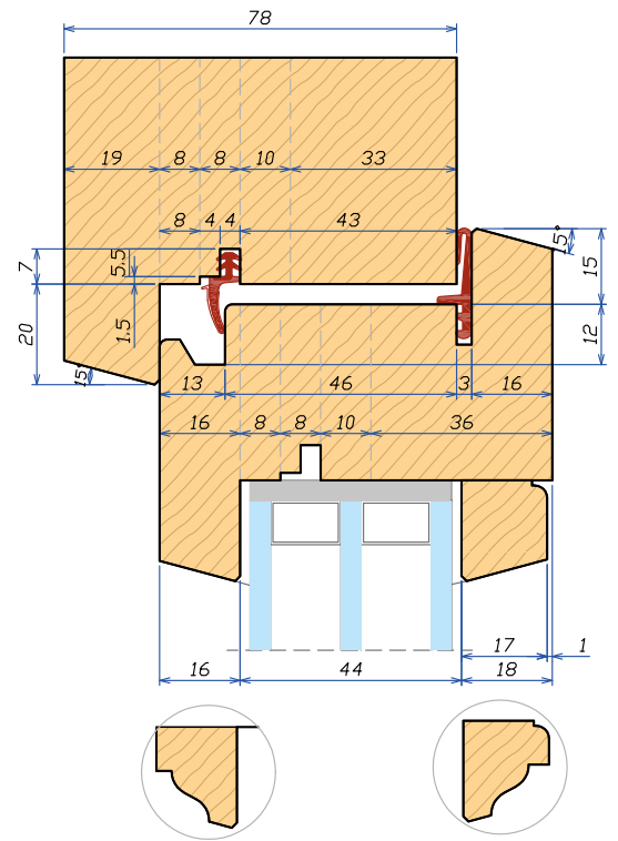
Sezione verticale 78 Vertical section 788
