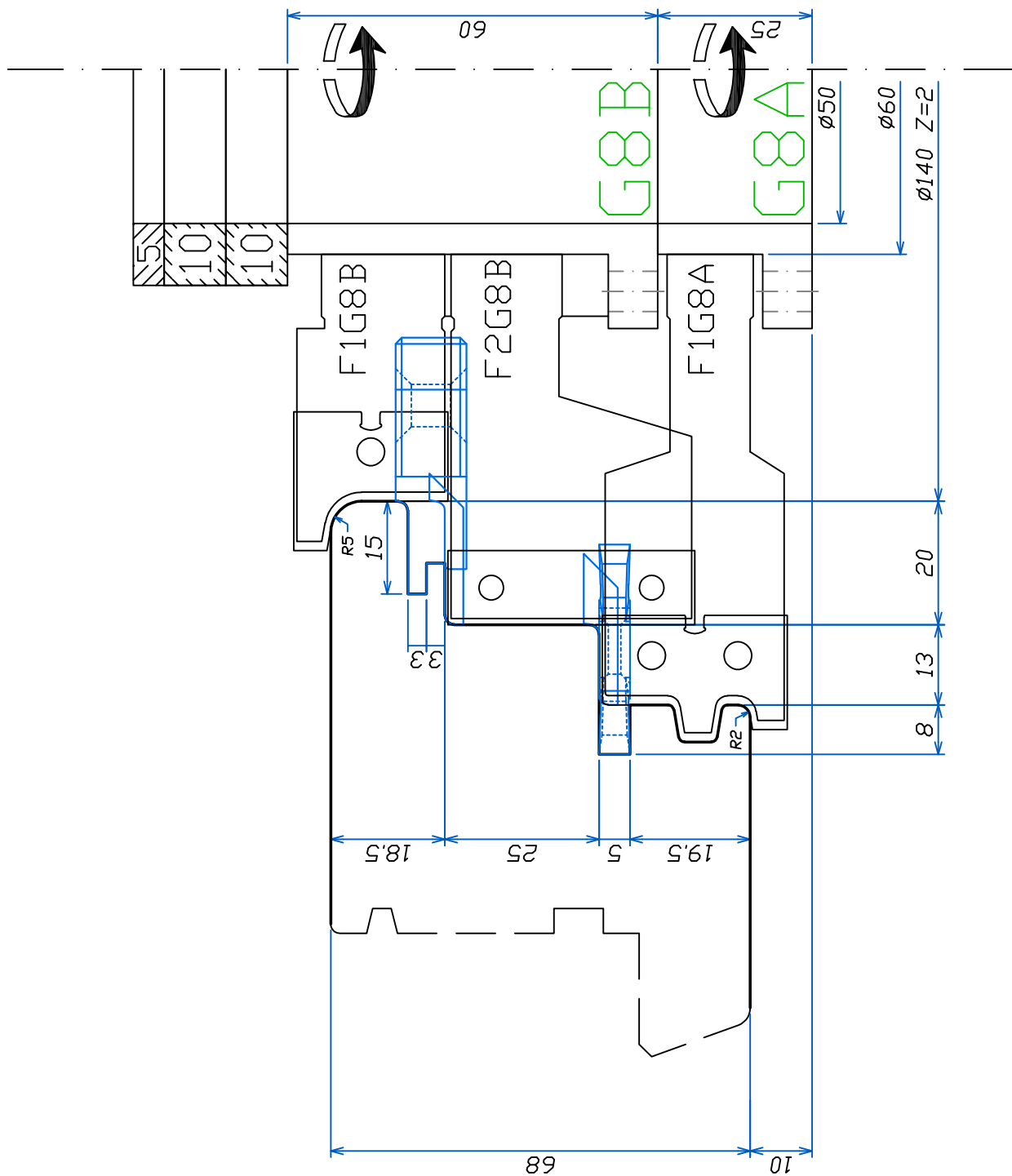
- EUROPRO CALIBRAGE OUVRANT 68 -
