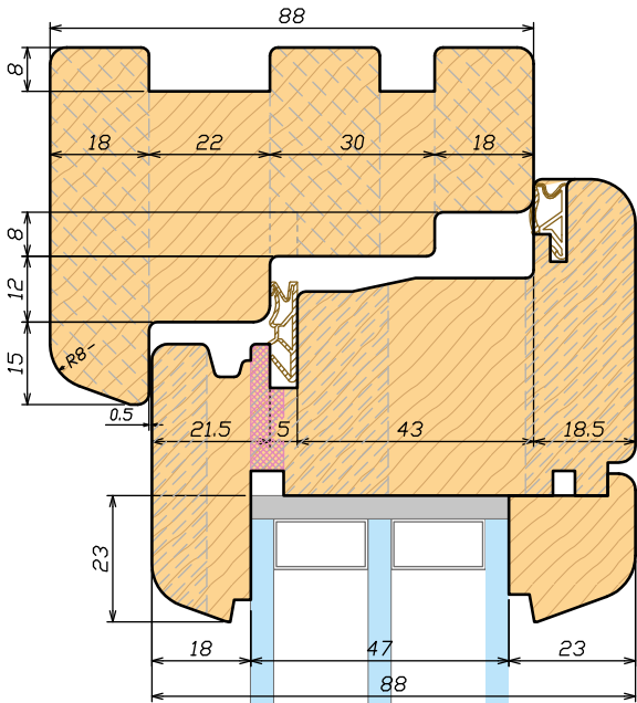
Sezione verticale 88 Vertical section 88
