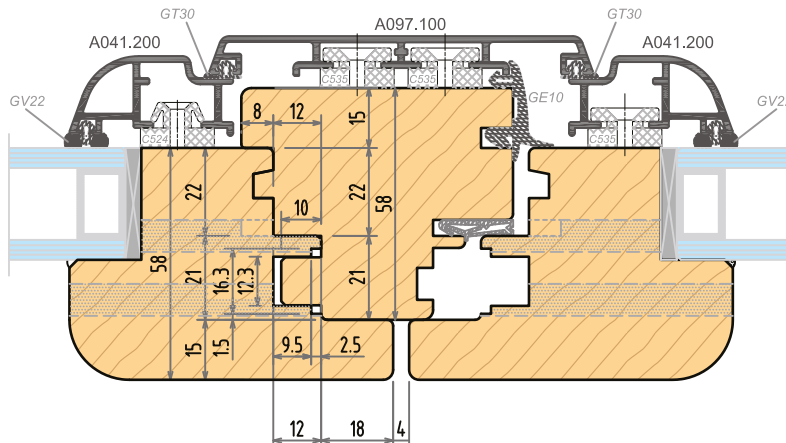
Sezione orizzontale chiusura centrale montantino aggiuntivo Horizontal section central closure additional jamb
