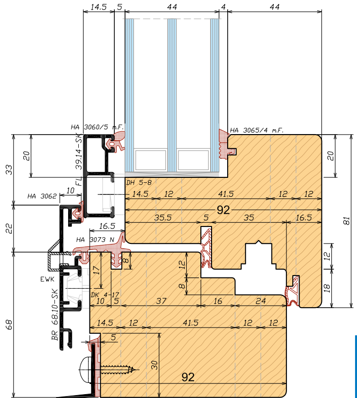
Sezione verticale Vertical section
