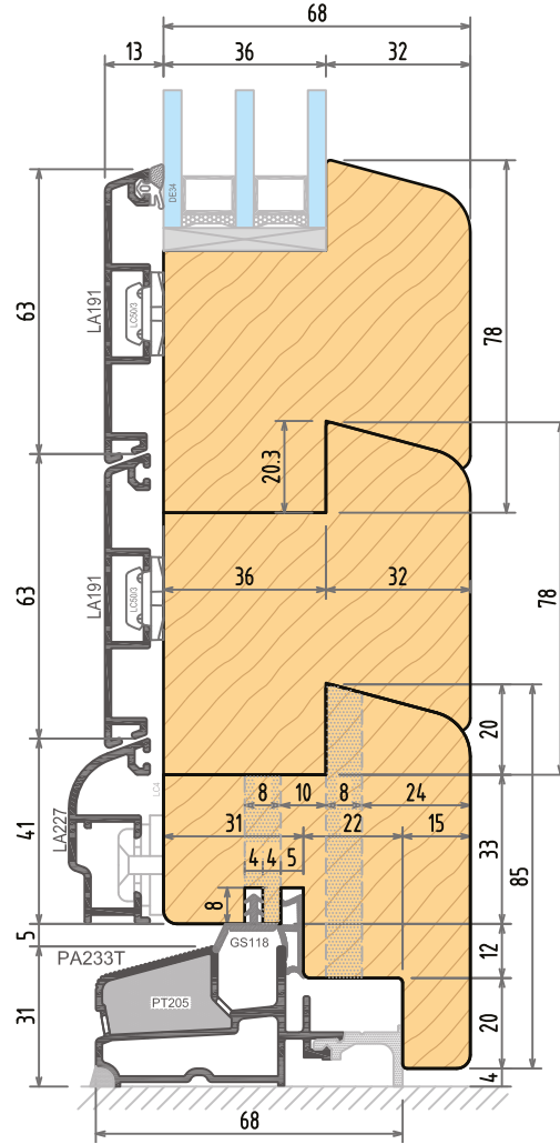
Sezione verticale - Portafinestra Vertical section - French door
