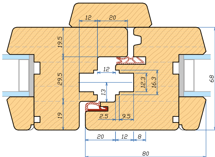
Sezione orizzontale - Chiusura centrale Horizontal section - Central closure
