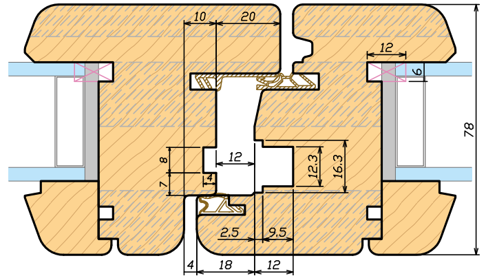
Sezione orizzontale - Chiusura centrale 78 Horizontal section - Central closure 78
