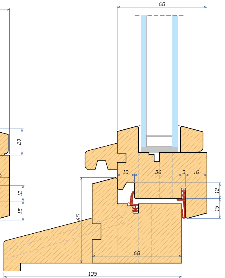
Sezione verticale 68 Vertical section 68
