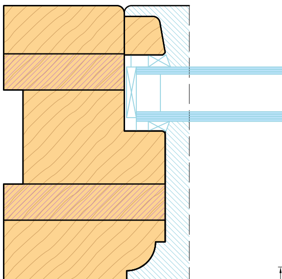
Sezione orizzontale Horizontal section
