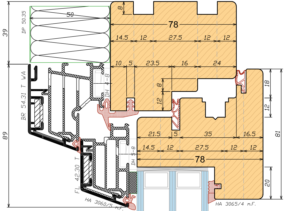
Sezione verticale Vertical section
