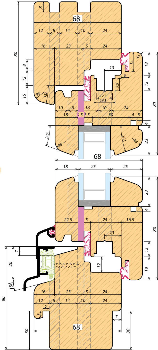
Sezione verticale Vertical section
