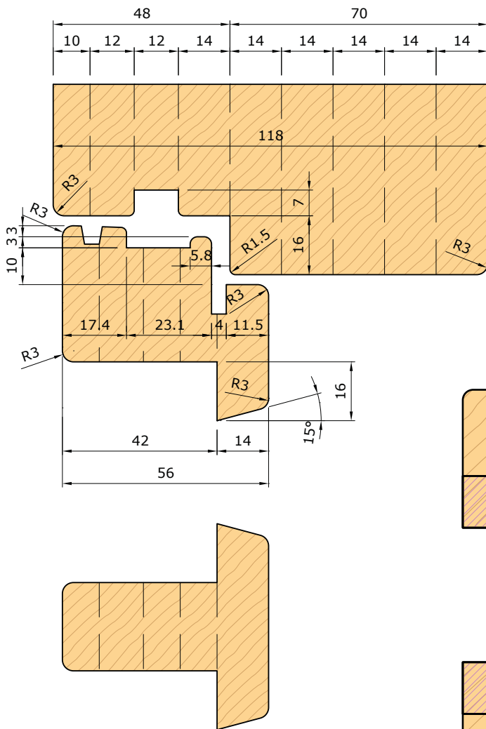
Sezione verticale Vertical section
