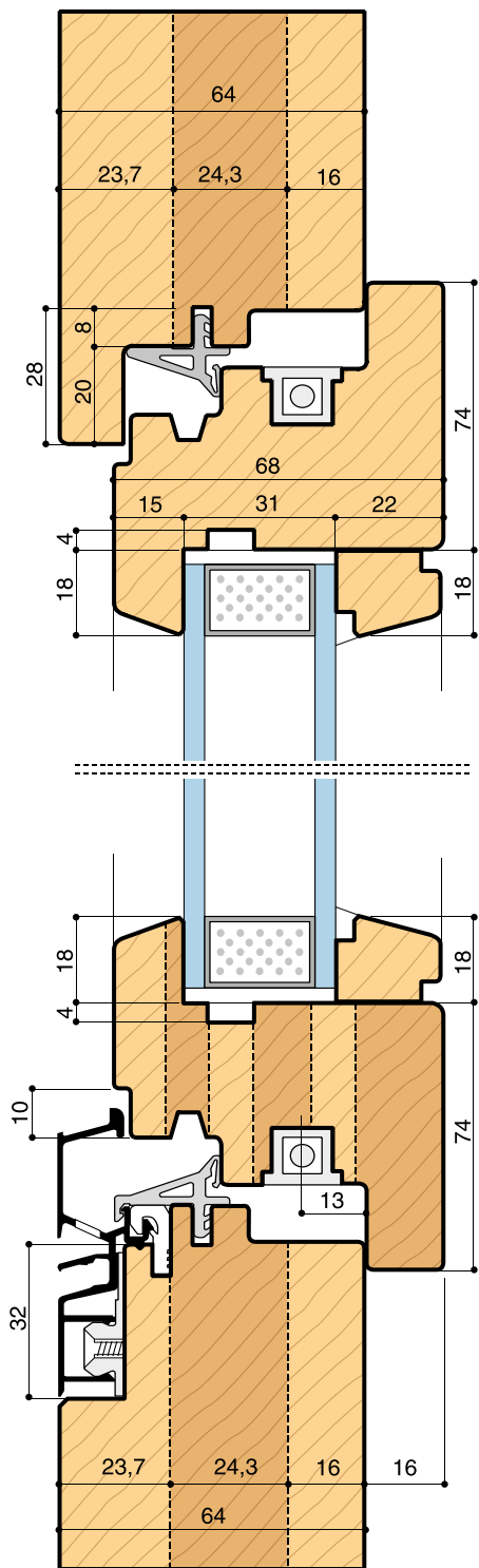
Sezione verticale Vertical section
