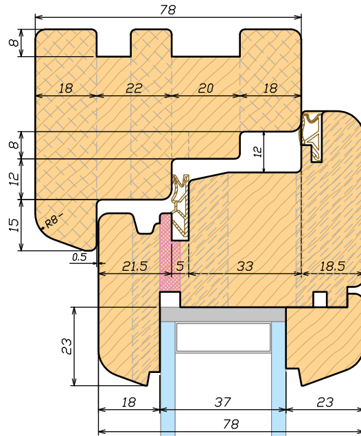
Sezione verticale 78 Vertical section 78
