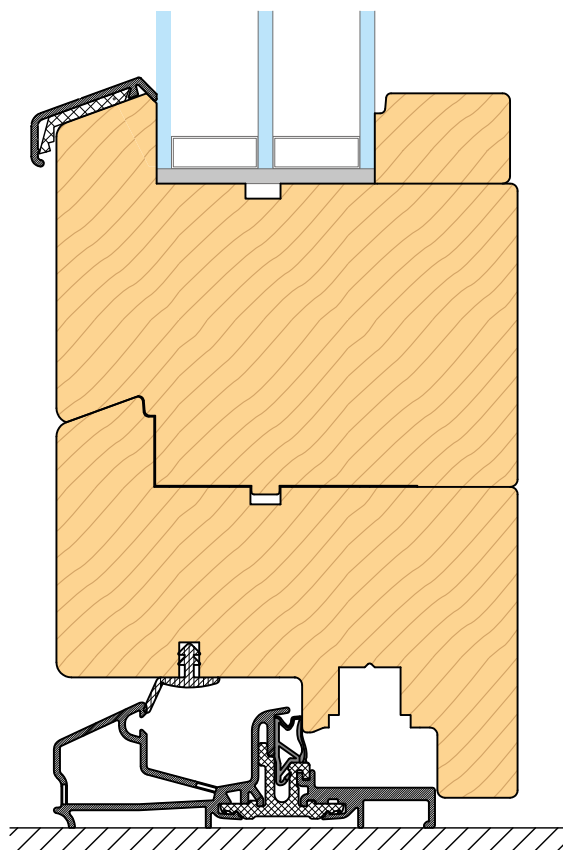
Sezione verticale - Portafinestra Vertical section - French door
