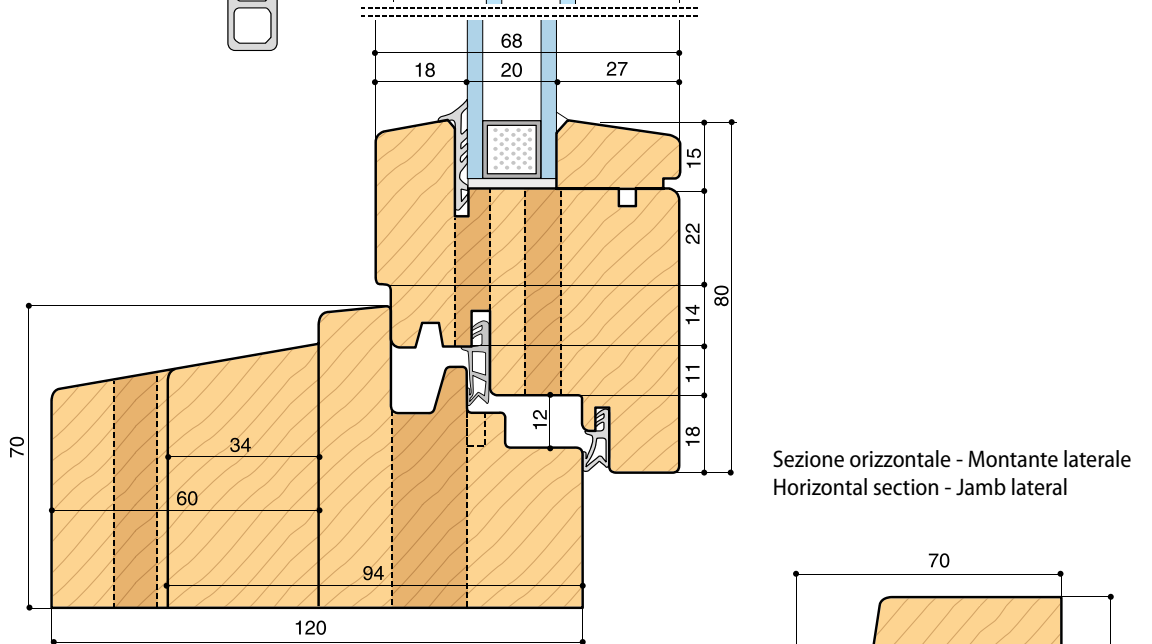
Sezione orizzontale - Chiusura centrale Horizontal section - Central closure
