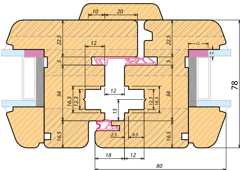
Sezione orizzontale - Chiusura centrale Horizontal section - Central closure
