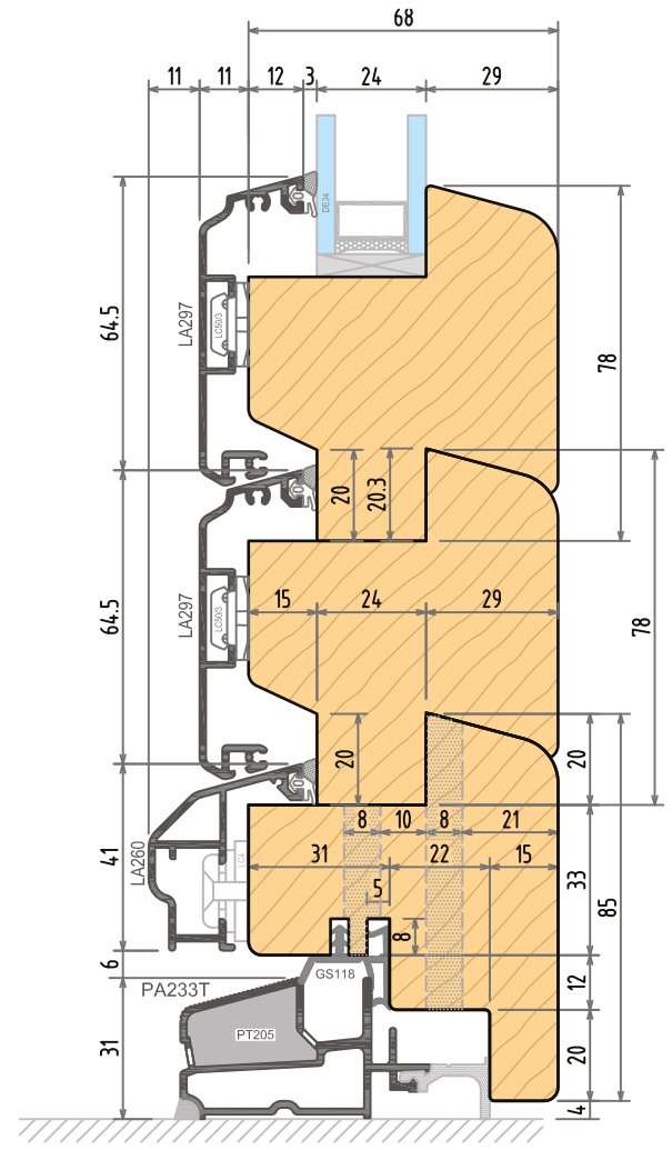
Sezione verticale - Portafinestra Vertical section - French door
