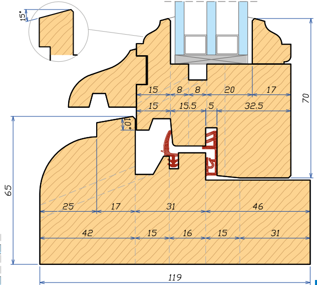
Sezione verticale Vertical section
