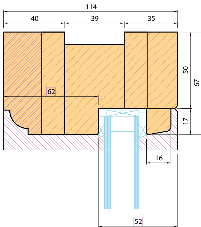
Sezione verticale Vertical section
