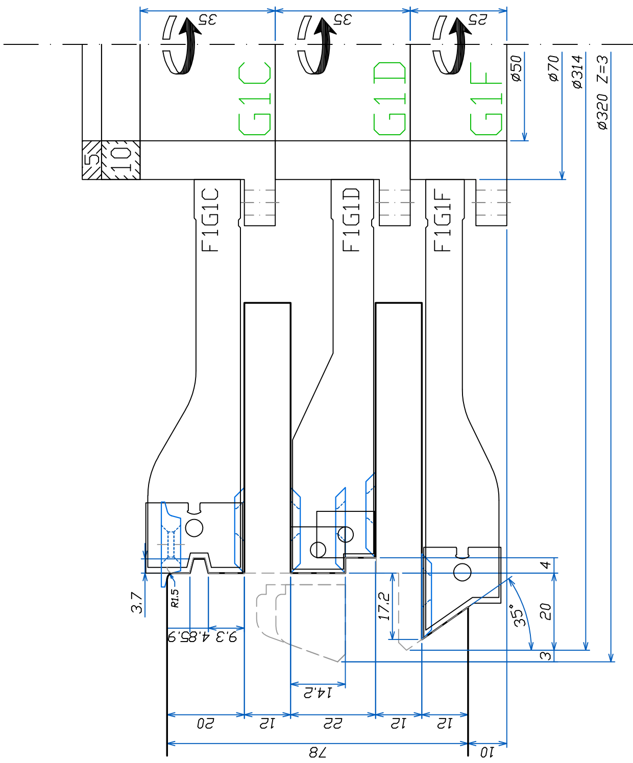
- EUROPRO TENONNAGE OUVRANT 78 35° -
