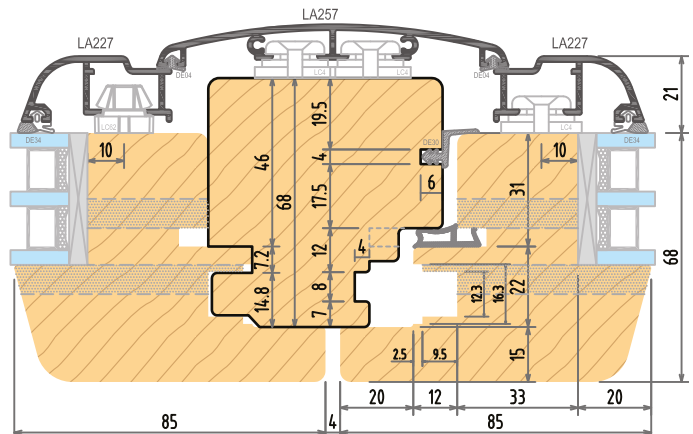
Montantino aggiuntivo Additional jamb
