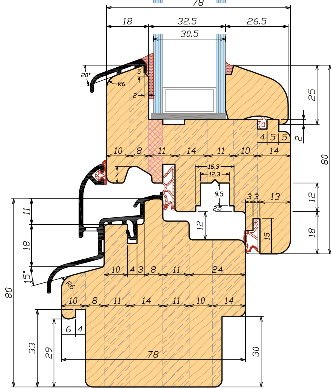
Sezione orizzontale - Chiusura centrale 78 Horizontal section - Central closure 78
